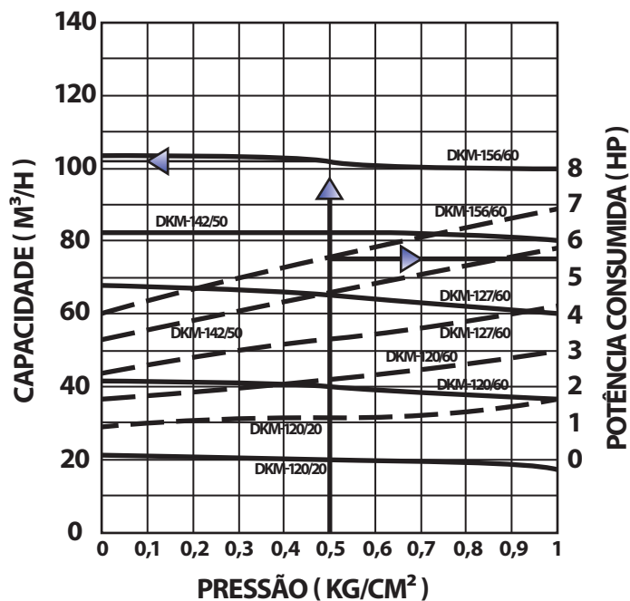
COMPRESSOR DE ANEL LÍQUIDO DOSITEC SÉRIE DKM
